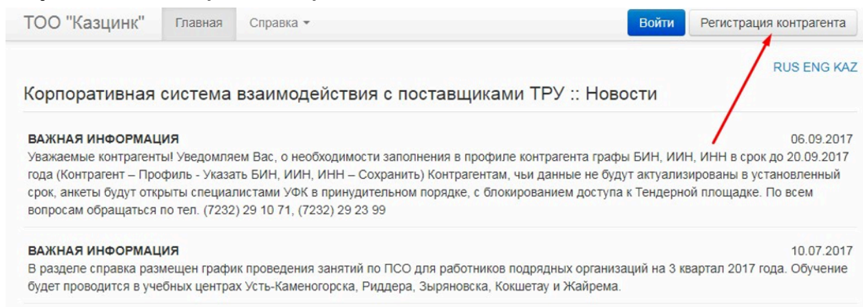
Рисунок 1.2.1. Регистрация контрагента.
